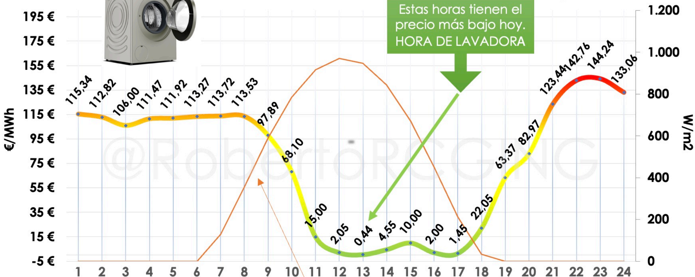
Curva SOLAR (FOTOVOLTAICA) del mes de AGOSTO en VALENCIA . Datos de Irradiancia global en cielo despejado en un plano fijo (W/m2)
